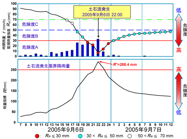
土石流災害発生と雨量指標 R' の相関図 (平成 17 年台風 14 号、宮島雨量観測所)
