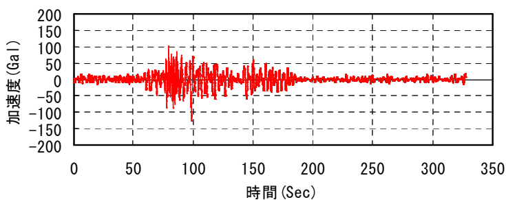
入力地震動の評価事例（時刻歴波形）
